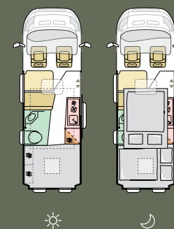
600 SX
